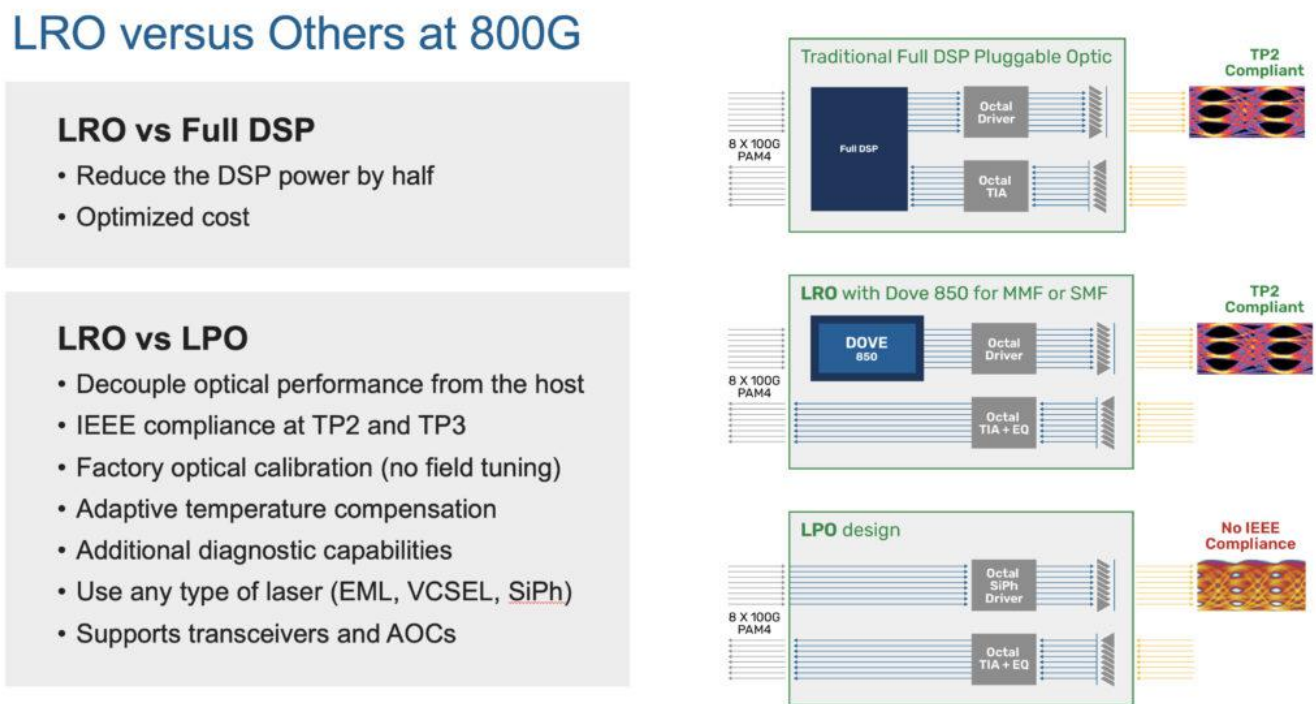
图 1：LRO 与 FULL DSP 和 LPO 对比
