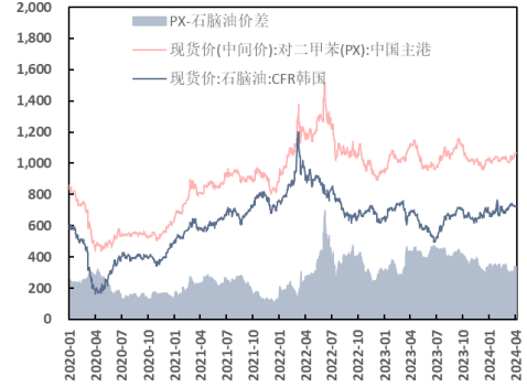
图 40: 石脑油、PX 价格及价差 (美元/吨)
