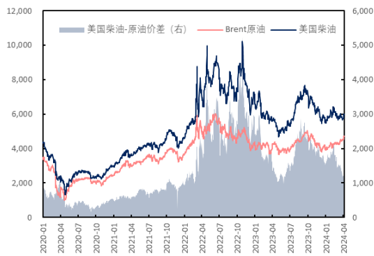
图 15: 原油、美国柴油价格及价差 (元/吨, 元/吨)
