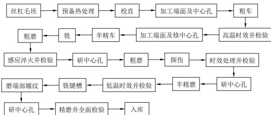
图：行星滚柱丝杠工艺流程图（丝杠）
