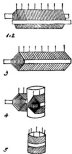
图：空心杯电机半卷绕式（左）和一次成型自动化绕制（右）
