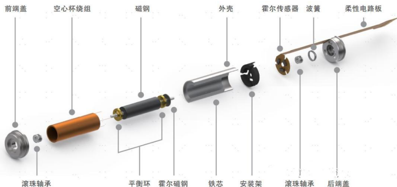
图：空心杯电机示意图
