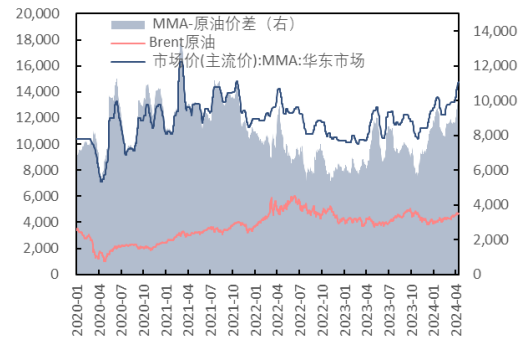
图 38: 原油、MMA 价格及价差 (元/吨, 元/吨)
