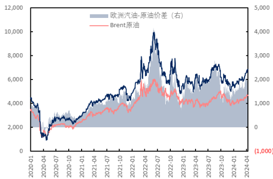
图 23: 原油、欧洲汽油价格及价差 (元/吨, 元/吨)
