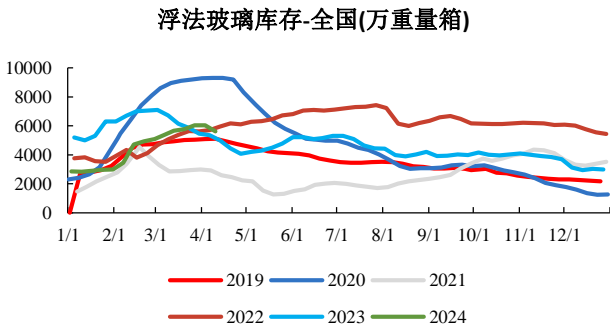
图36: 全国浮法玻璃库存接近 2022 年同期水平
