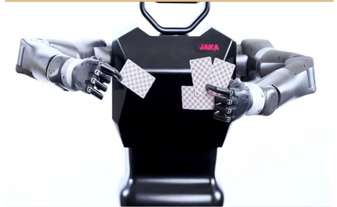
图 7：K-1 可以完成抓扑克的精细动作
