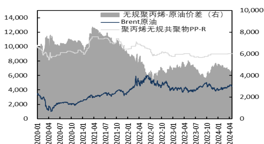
原油、无规聚丙烯价格及价差 (元/吨, 元/吨)
