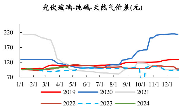
图52: 当前光伏玻璃盈利能力位于2021年同期水平
