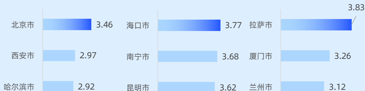
公交&地铁出行意愿指数
