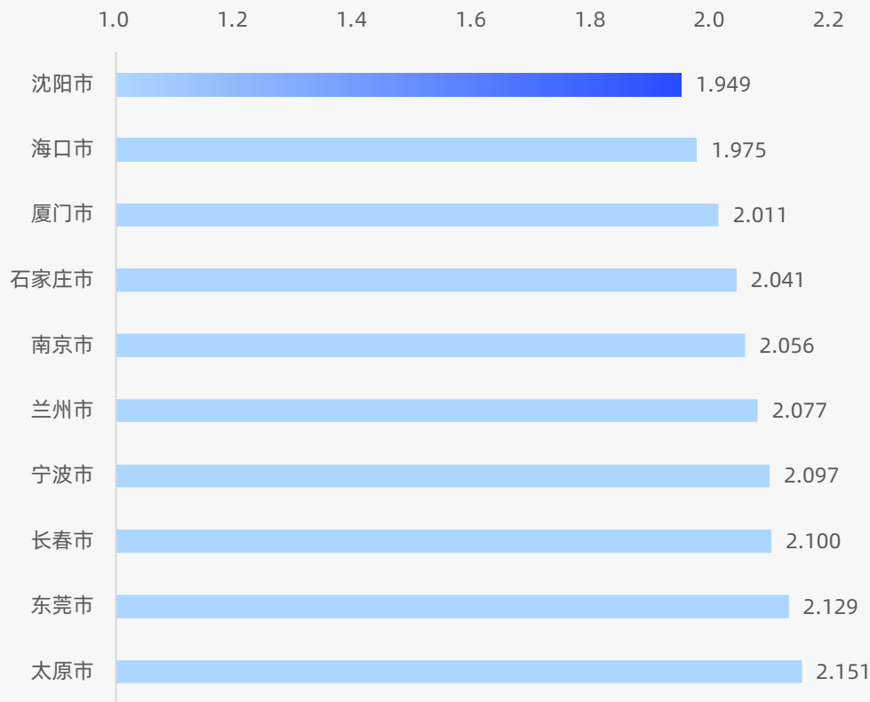
高峰社会车辆-公交车速比
