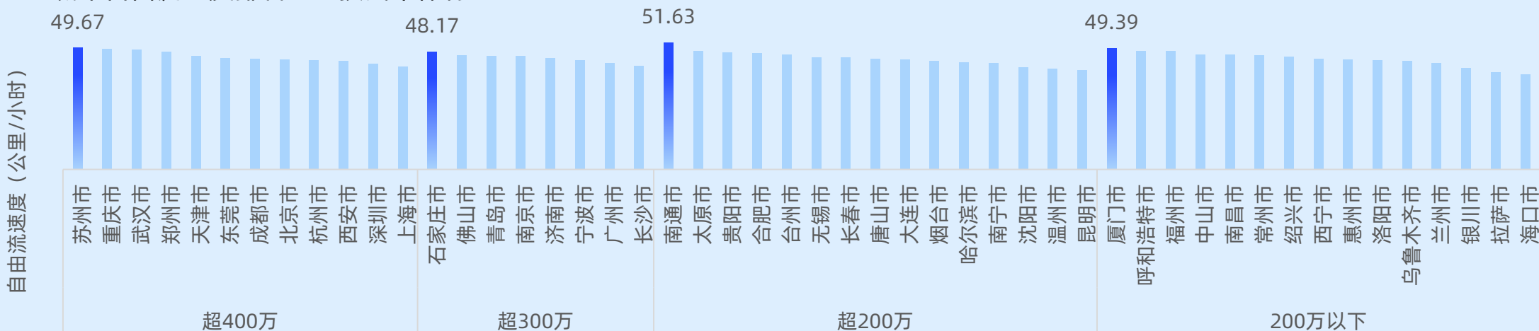
50城市自由流速度排名——按汽车保有量
