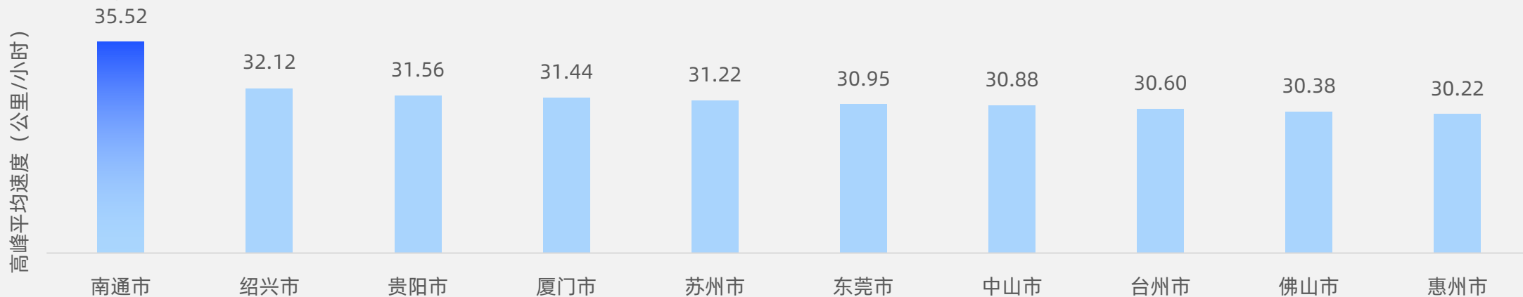
城市高峰平均车速排名TOP10
