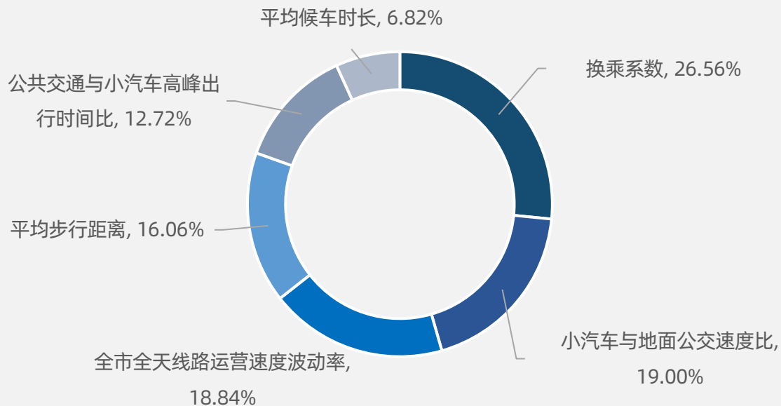
六项指标信息熵权重分配
