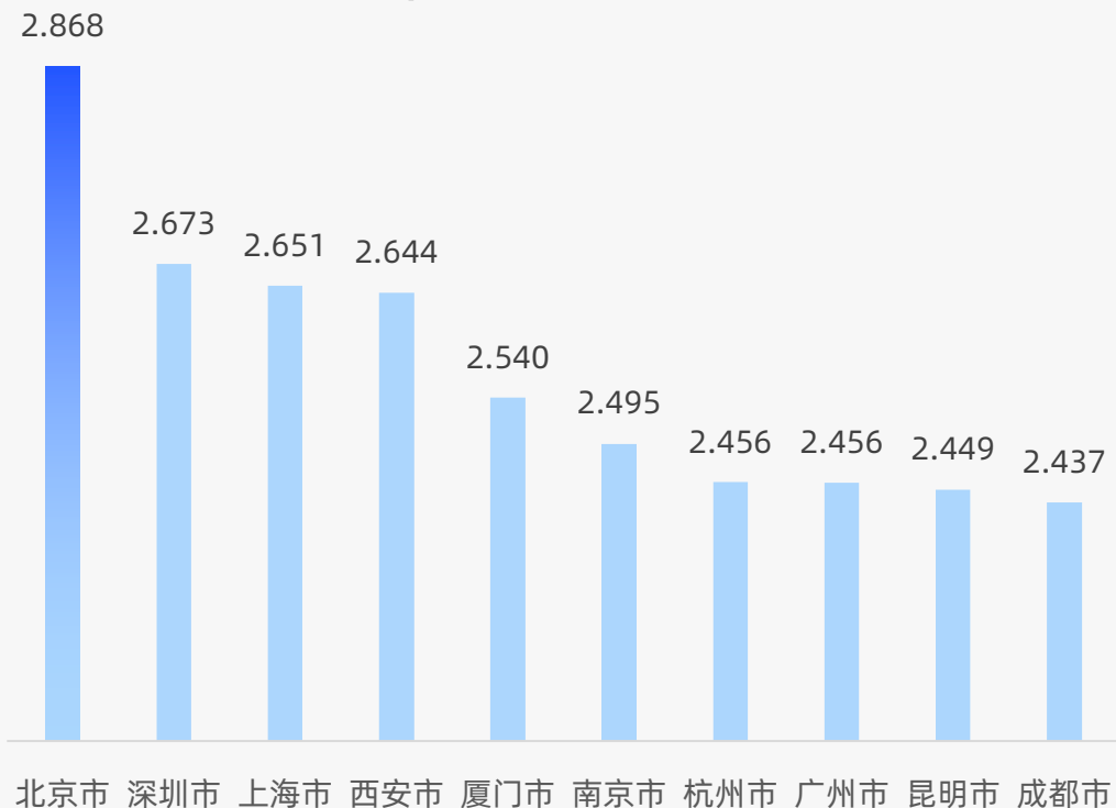
2024Q1绿色出行意愿指数TOP10
