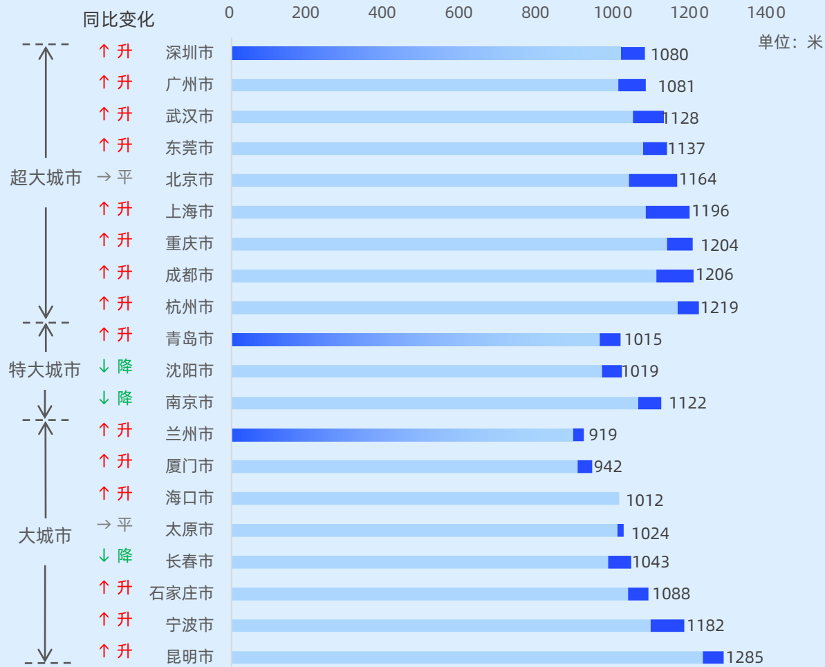
■ 进出公交系统平均步行距离 ■ 平均换乘距离
