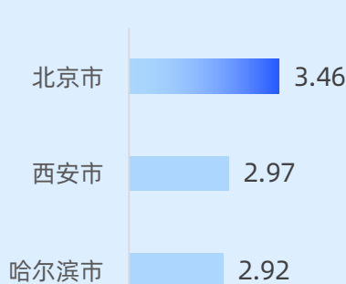
公交&地铁出行意愿指数
