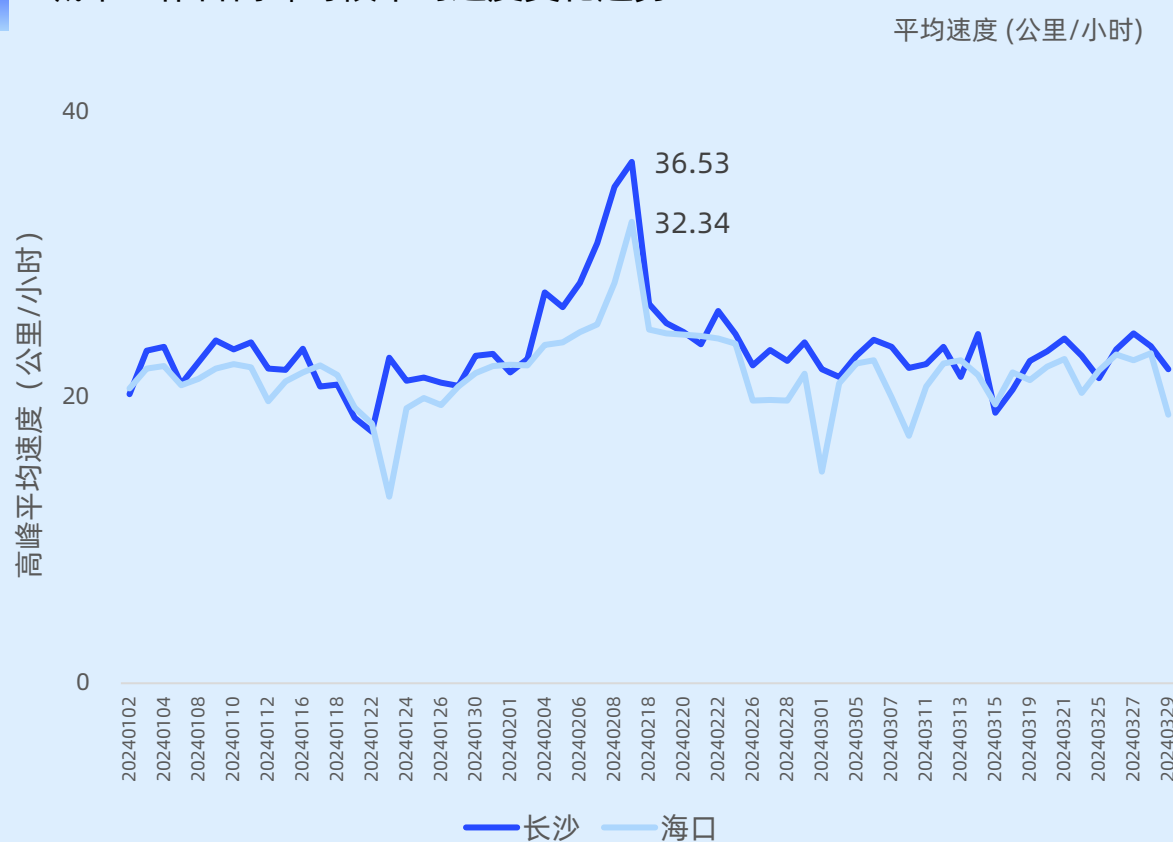
城市工作日高峰时段平均速度变化趋势
