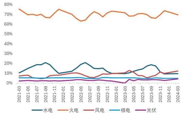
图 13：3 月分类型发电量占比
