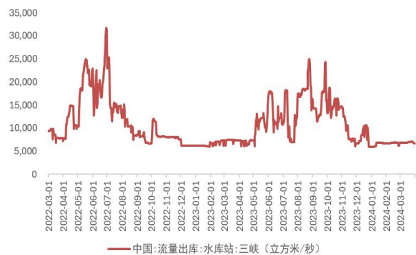
图 48：三峡出库流量日行情（立方米/秒）
