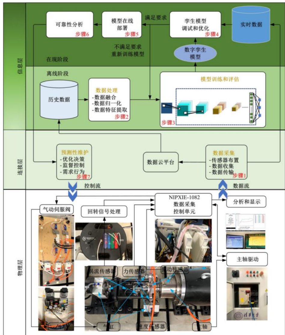
图表33: 基于数字孪生的数控机床可靠性分析信息物理融合系统框架
