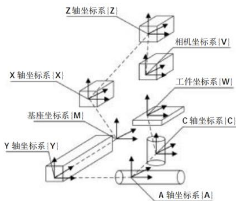
图表29: 加入视觉系统后的五轴机床关键部件固联坐标系
