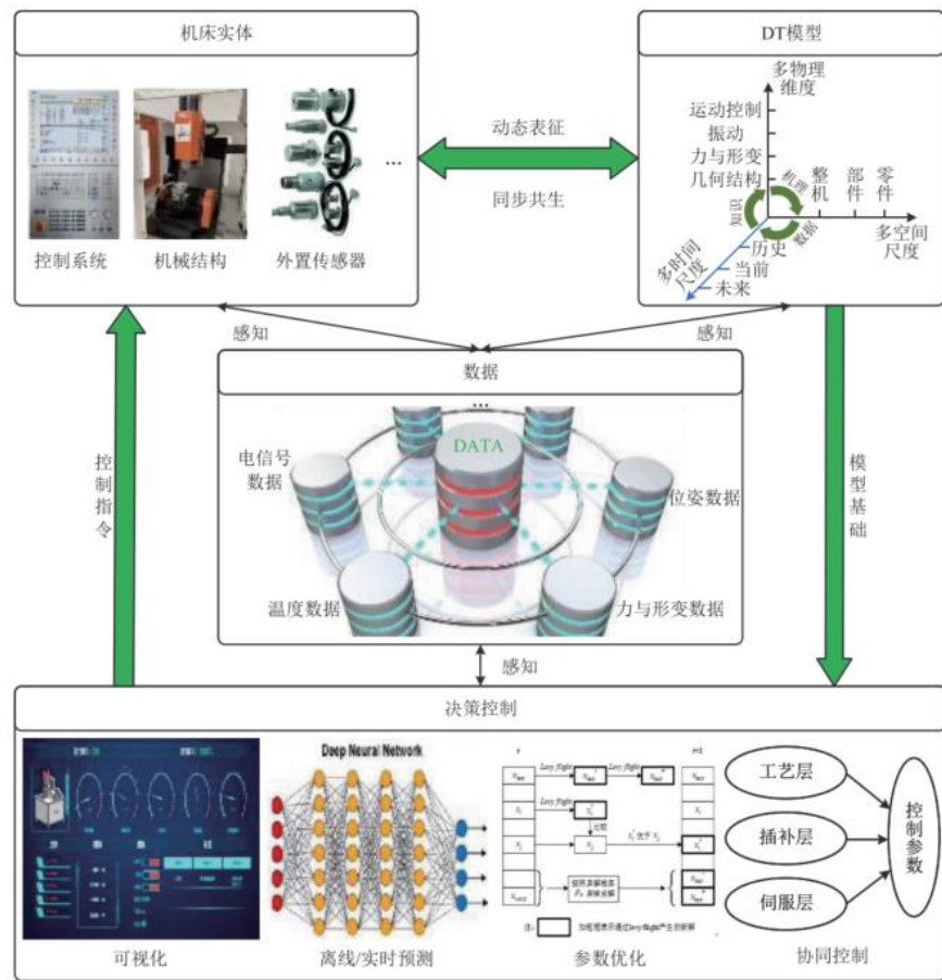
图表32: 数字孪生机床体系架构
