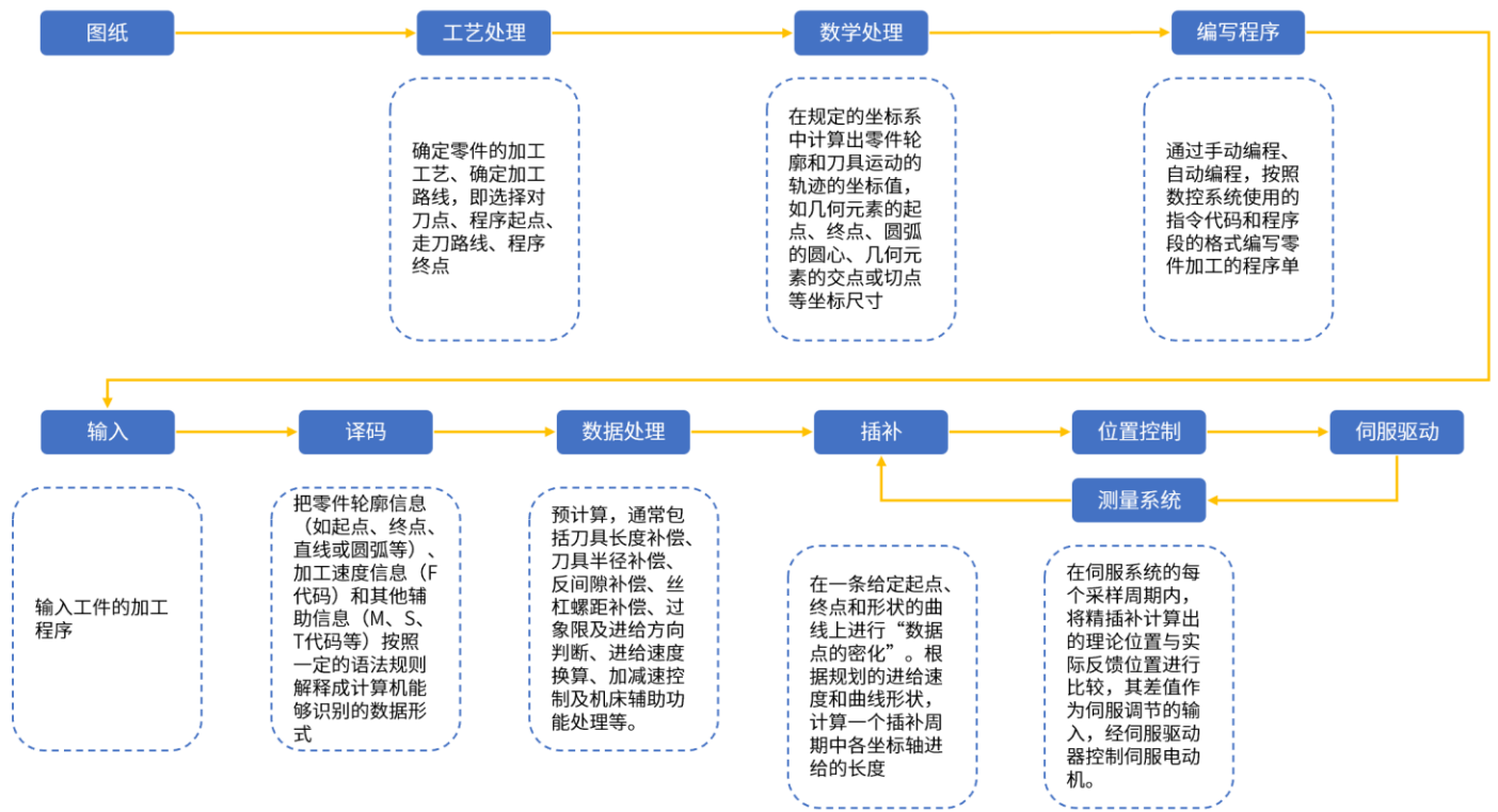
图表17: 数控系统控制原理
