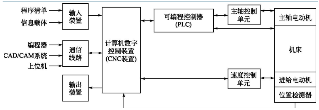
图表15: CNC 系统组成
