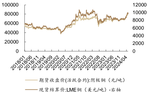
图 11：本周 SHFE 铜价下跌 0.4%,LME 铜价上涨 2.1%
