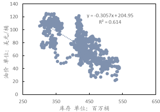
图 36: 2010-2024.05 美国商业原油库存与油价相关性
