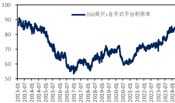
图 18：350 英尺+自升式钻井平台利用率 (%)
