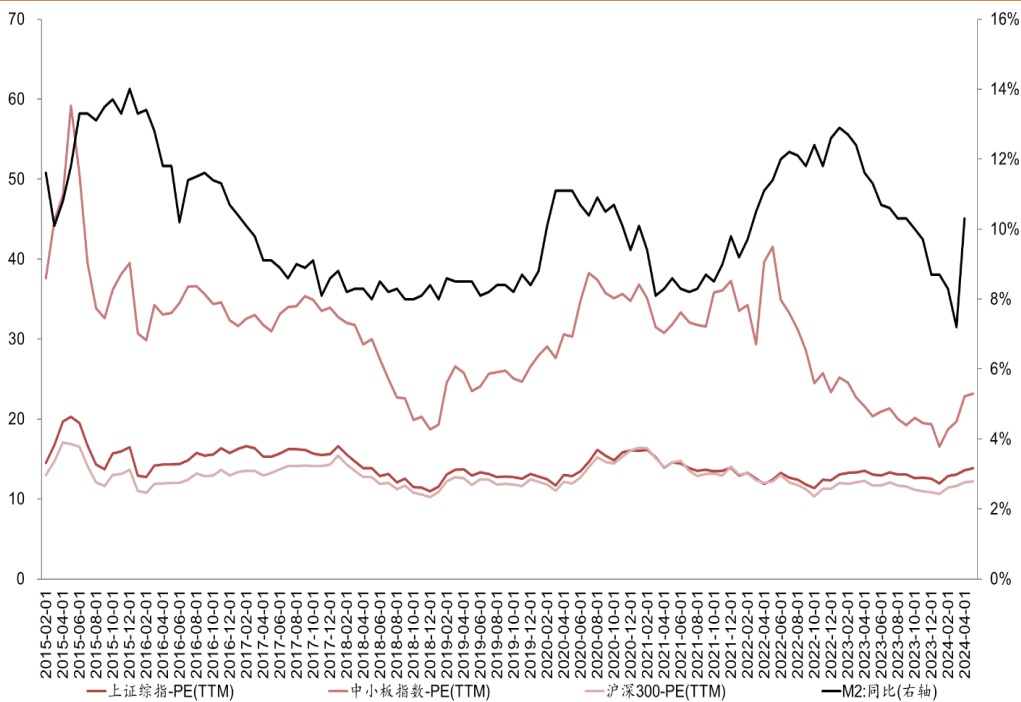
图 12: 2015 年至今的 M2 同比数据与股指市盈率的关系
