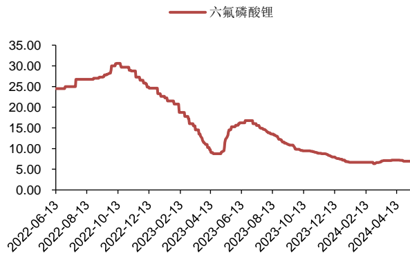
图 30: 六氟磷酸锂价格走势 (万元/吨)
