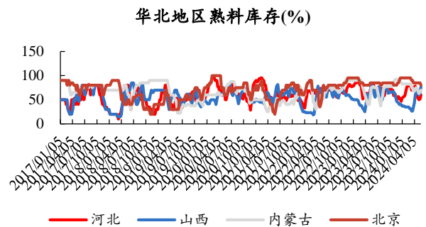
图13: 本周华北地区熟料库存北京环比下降, 河北、山西、内蒙古环比上升
