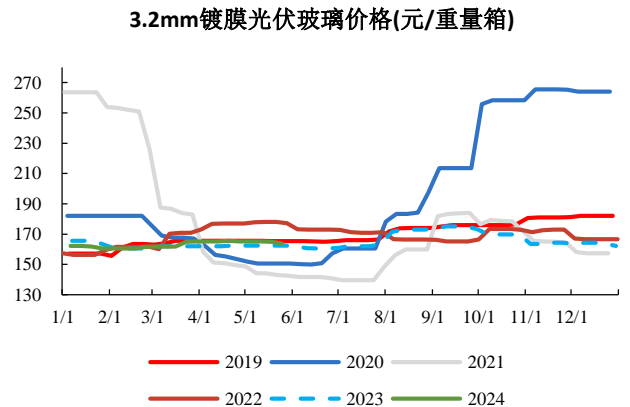
图39：当前光伏玻璃价格接近2023年同期水平
