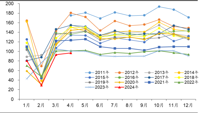
图12 挖机开挖小时数（小时）
