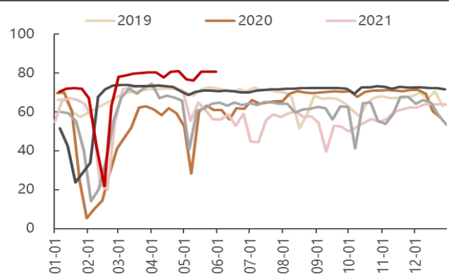
图12：汽车轮胎（半钢胎）开工率微降 (%)
