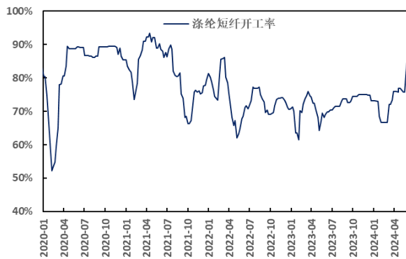
图 59: 2020-2023 年涤纶短纤开工率 (%)
