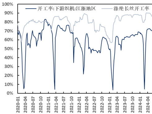
图 51: 涤纶长丝与下游织机开工率 (%)
