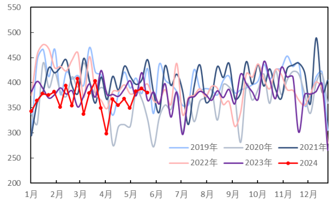
图 65: 美国柴油消费量 (万桶/天)
