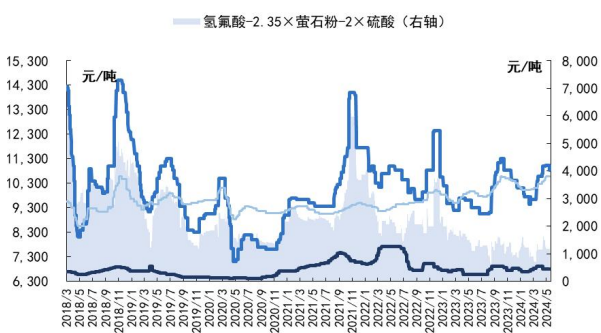
图5：萤石-氢氟酸价格与价差走势
