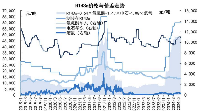
图10：三代制冷剂 R143a 价格与价差走势
