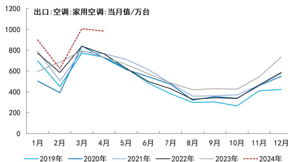
图55: 我国家用空调出口数据季节图-月度
