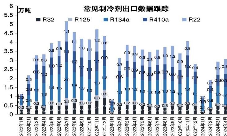
图13：2022-2023 年各主要制冷剂出口量趋势
