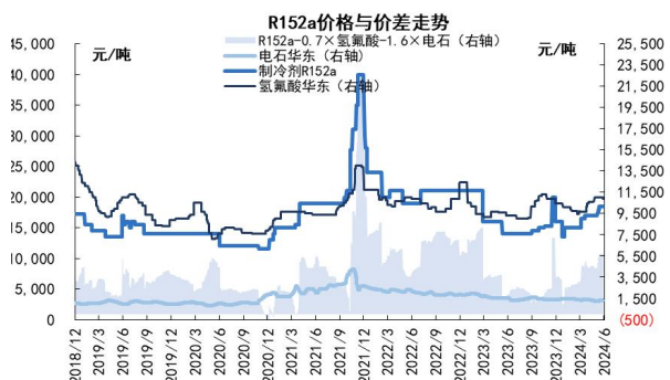
图11：三代制冷剂 R152a 价格与价差走势
