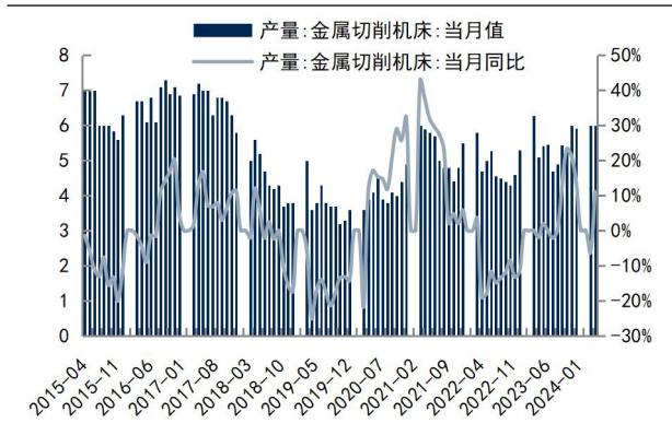
图19：2024年4月金属切削机床产量同比增长11.10%
