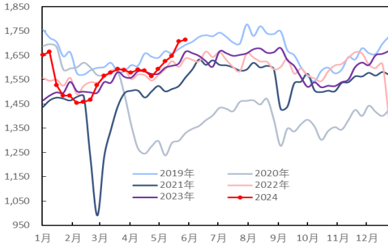
图 30: 美国炼厂原油加工量 (万桶/天)
