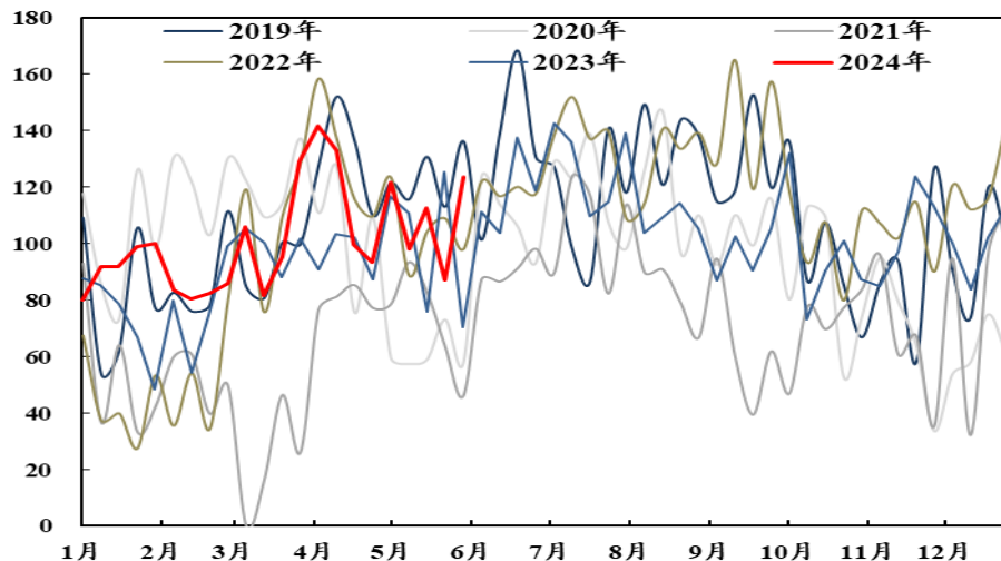
美国柴油净出口量 (万桶/天)
