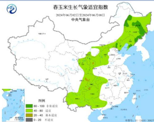
图10：春玉米生长气象适宜指数（6.2-6.8）
