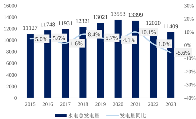
图13: 2015-2023 年水电发电量 (亿千瓦时)
