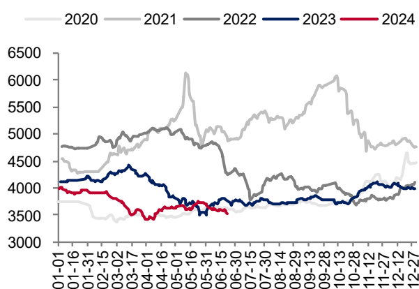
图表 54: 价格:螺纹钢:HRB400 20mm:上海
