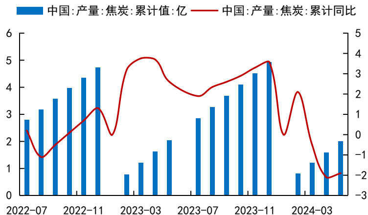
图28 焦炭累计产量及同比增速（亿吨，%）
