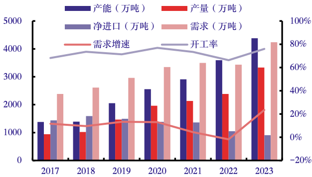
图14: 我国对二甲苯 (PX) 供需统计
