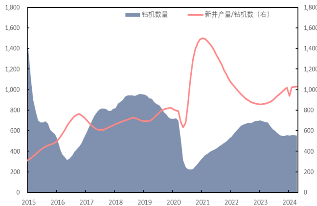
图 60: 美国七大页岩油产区总钻机数量和平均单个钻机对应的的新井原油产量 (台, 桶/日)
