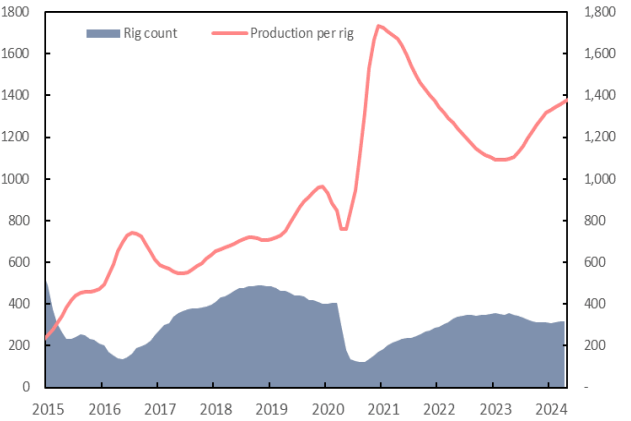
图 61: 美国 Permian 产区钻机数量和单个钻机对应的的新井原油产量 (台, 桶/日)
