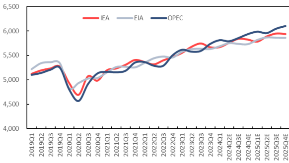
图 73: IEA、EIA、OPEC 对 2019-2025 年非 OECD 国家原油需求及预测季度数据 (万桶/日)
