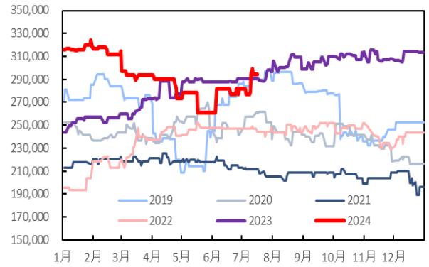
图 15: 8000 英尺+半潜式钻井平台平均日费 (美元/天)
