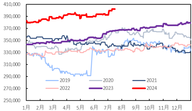
图 17: 8000 英尺+钻井船平均日费 (美元/天)
