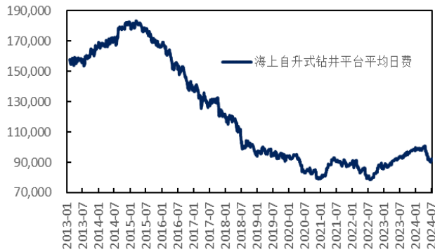
图 12: 350 英尺+自升式钻井平台平均日费 (美元/天)
