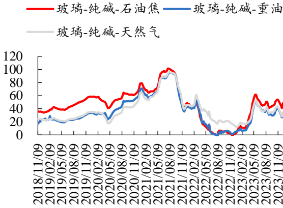
图47：本周浮法玻璃盈利下跌
