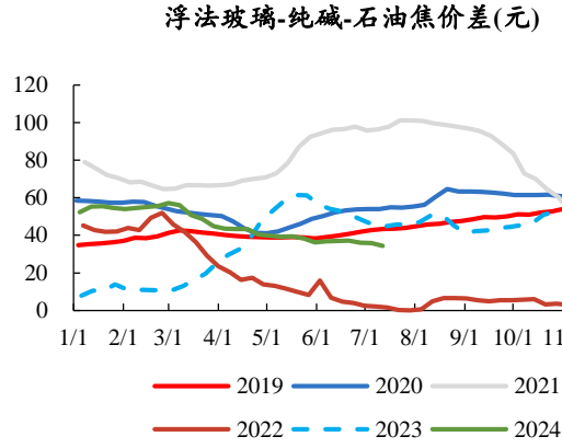
图48：本周浮法玻璃-纯碱-石油焦价差下跌
