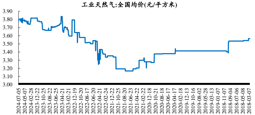
图46：本周全国工业天然气价格环比上涨 1.04%
