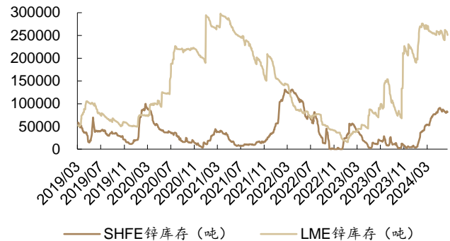
图 29：本周 SHFE 锌库存增加 1.6%,LME 锌库存减少 2.9%
