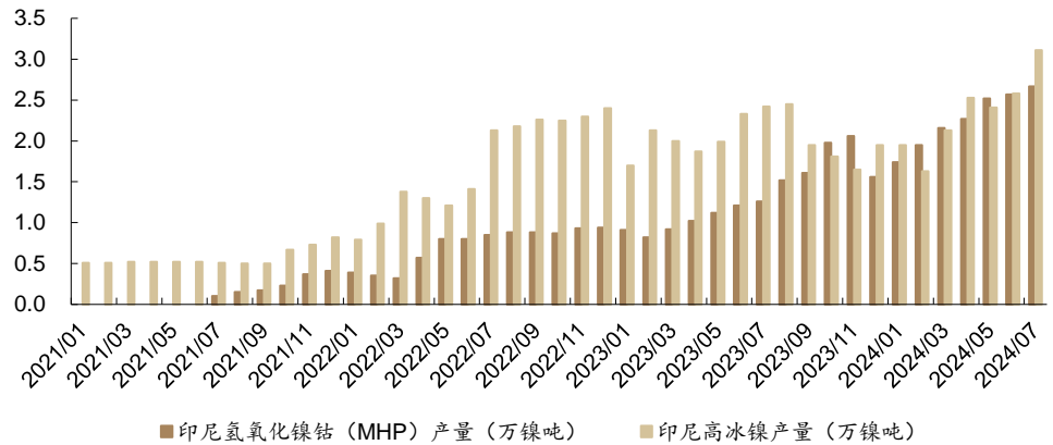
图 53: 2024 年 7 月, SMM 预计印尼氢氧化镍钴 (MHP) 产量 2.67 万镍吨, 印尼高冰镍产量 3.11 万镍吨
