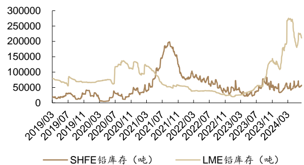
图 24：本周 SHFE 铅库存增加 5.2%，LME 铅库存减少 4.8%
