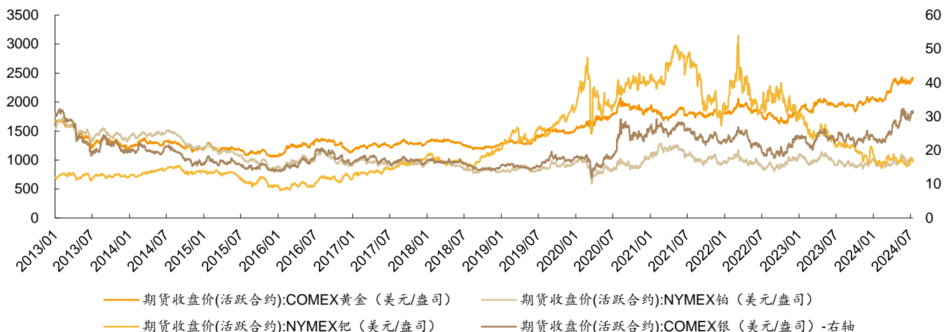
图 2：截至 2024 年 7 月 12 日，COMEX 银价格 31.0 美元/盎司，周变动-1.6%；NYMEX 铂价格 1014.9 美元/盎司，周变动-2.8%；NYMEX 钯价格 970.0 美元/盎司，周变动-6.3%
