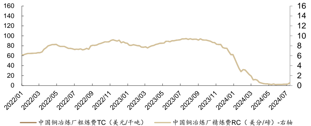
图 15: 截至 2024 年 7 月 12 日, 中国铜冶炼厂粗炼费 TC5.50 美元/千吨; 中国铜冶炼厂精炼费 RC0.55 美分/磅
