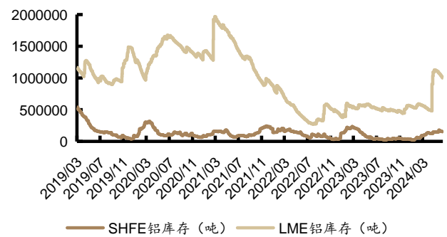
图 18: 本周 SHFE 铝库存减少 2.4%,LME 铝库存减少 2.3%
