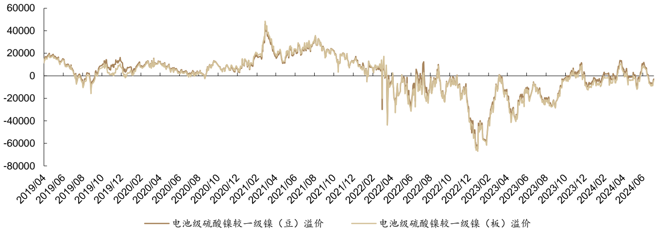
图 50: 截至 2024 年 7 月 12 日, 电池级硫酸镍较一级镍(豆)溢价-2891 元/镍吨, 电池级硫酸镍较一级镍(板)溢价-4266 元/镍吨
