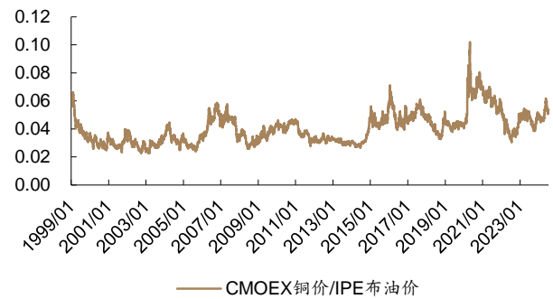
图 14: 截至 2024 年 7 月 12 日, COMEX 铜价/IPE 布油价 0.0537
