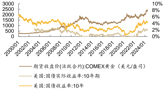
图 3:截至 2024 年 7 月 12 日,美国十年期国债实际收益率 1.94%
