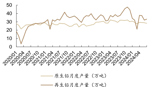
图 26：2024 年 6 月，再生铅月度产量 33 万吨，同比减少 8.95%，2024 年 6 月，原生铅月度产量 28 万吨，同比减少 3.55%
