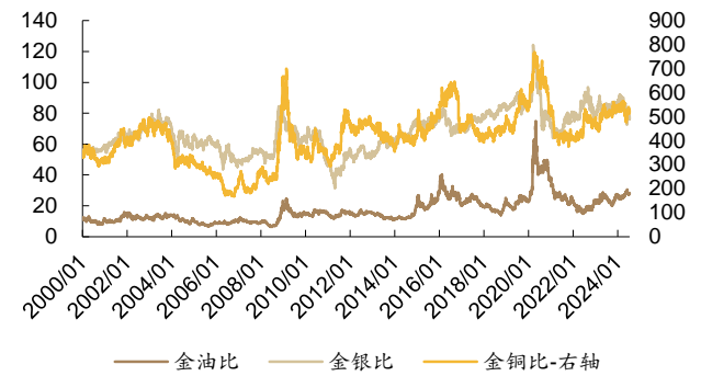
图 6:2024 年 7 月 12 日,金油比 28.33,金银比 77.87,金铜比 527.40
