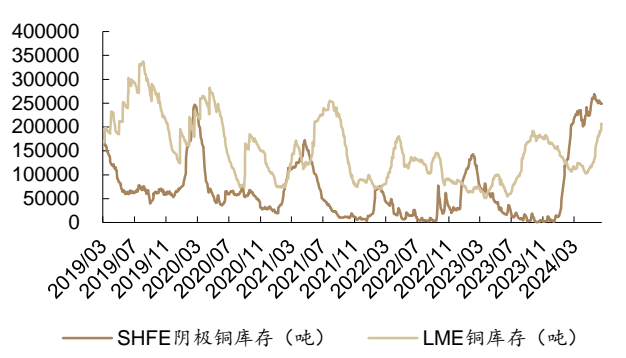
图 12：本周 SHFE 铜库存减少 0.8%,LME 铜库存增加 7.6%
