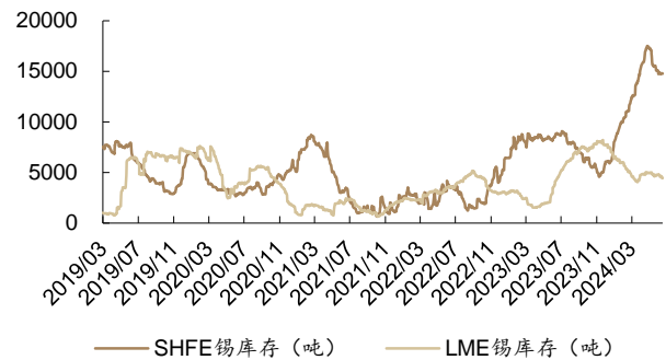
图 34：本周 SHFE 锡库存增加 0.1%,LME 锡库存减少 2.8%
