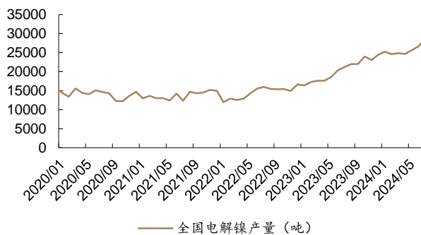
图 40: 2024 年 6 月, 全国电解镍产量 26650 吨, 同比增加 30.77%
