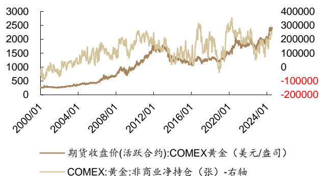
图 10：2024 年 7 月 9 日，COMEX:黄金:非商业净持仓 254775 张
