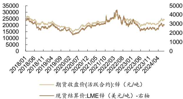
图 28：本周 SHFE 锌价下跌 2.01%,LME 锌价下跌 2.9%
