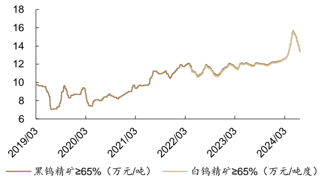
图 42: 截至 2024 年 7 月 12 日, 黑钨精矿 ( \geq 65\% ) 13.45 万元/吨, 下跌 2.9%; 白钨精矿 ( \geq 65\% ) 13.35 万元/吨, 下跌 2.9%
