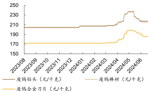
图 43: 截至 2024 年 7 月 12 日, 废钨钻头 216 元/千克, 持平; 废钨棒材 218 元/千克, 持平; 废钨合金刀片 183.50 元/千克, 下跌 1.1%
