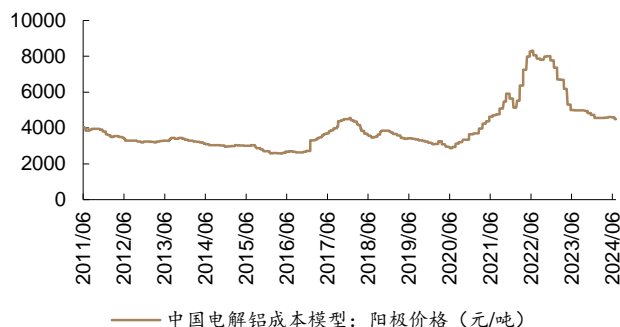
图 21: 截至 2024 年 7 月 11 日, 阳极价格 4491 元/吨
