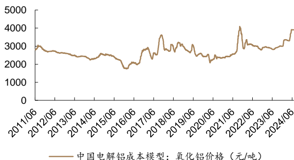
图 20: 截至 2024 年 7 月 11 日, 氧化铝价格 3903 元/吨
