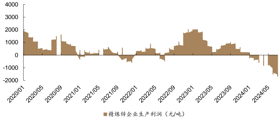
图 32：截至 2024 年 7 月 11 日，精炼锌企业生产利润-1638 元/吨
