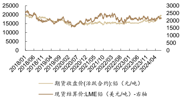
图 23：本周 SHFE 铅价下跌 1.0%，LME 铅价下跌 2.8%
