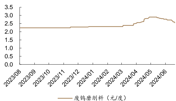
图 44: 截至 2024 年 7 月 12 日, 废钨磨削料 2.55 元/度, 下跌 6.3%
