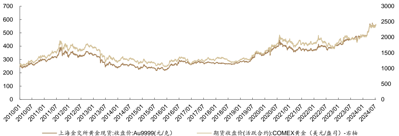
图 1：截至 2024 年 7 月 12 日，上海金交所黄金现货 Au9999 收盘价 563 元/克，周变动 0.9%；截至 2024 年 7 月 12 日，期货收盘价(活跃合约):COMEX 黄金 2416 美元/盎司，周变动 0.7%
