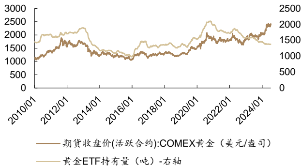
图 5:截至 2024 年 7 月 11 日,黄金 ETF 持有量 1377 吨
