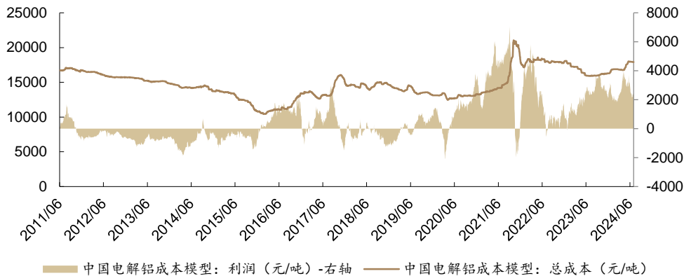
图 19: 截至 2024 年 7 月 11 日, 电解铝成本 17907 元/吨, 周变化 0.00%, 电解铝利润 2233 元/吨, 周变化-5.50%
