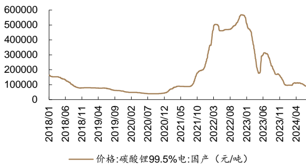
图 51: 本周碳酸锂:99.5%:电:国产 价格下降 0.9%
