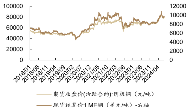
图 11：本周 SHFE 铜价下跌 1.8%,LME 铜价下跌 1.4%
