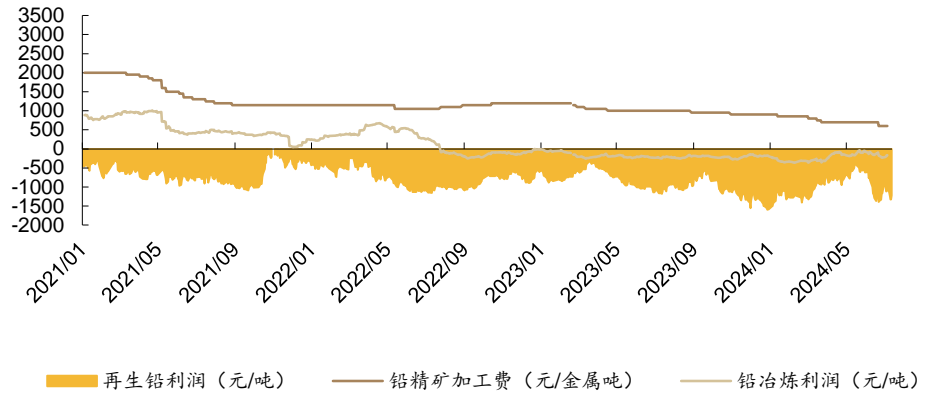
图 27：2024 年 7 月 5 日，铅精矿加工费 600 元/吨，铅冶炼利润-169 元/吨。2024 年 7 月 12 日，再生铅利润-1224 元/吨
