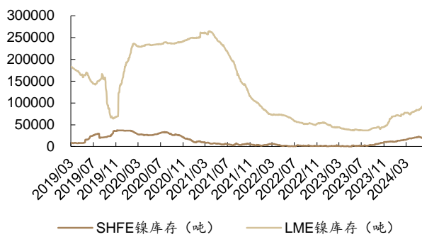
图 38: 本周 SHFE 镍库存减少 2.8%, LME 镍库存增加 1.3%
