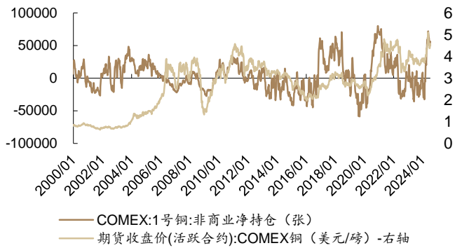
图 13: 截至 2024 年 7 月 9 日, COMEX:1 号铜:非商业净持仓 56031 张
