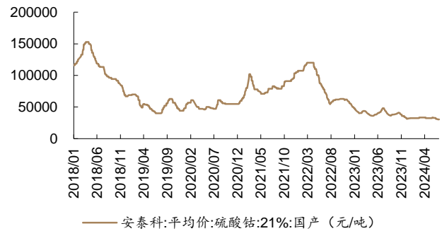
图 52: 本周硫酸钴:21%:国产 价格下降 0.2%
