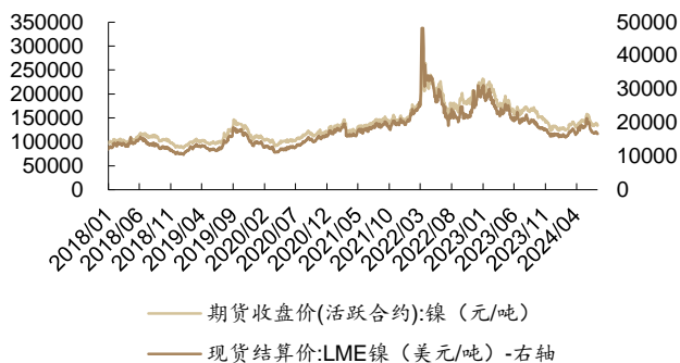
图 37: 本周 SHFE 镍价下跌 2.2%, LME 镍价下跌 3.2%
