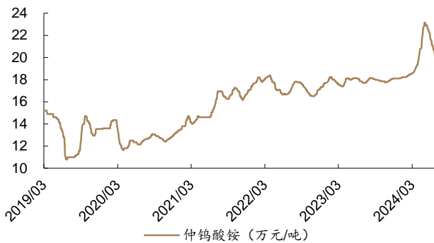
图 41: 截至 2024 年 7 月 12 日, 仲钨酸铵 20.30 万元/吨, 环比下跌 1.9%
