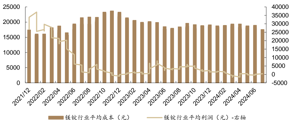
图 47：2024 年 7 月 5 日，镁锭行业平均成本 17567 元/吨，镁锭行业平均利润 363 元/吨
