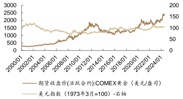
图 4:截至 2024 年 7 月 12 日,美元指数(1973 年 3 月=100)为 104.10
