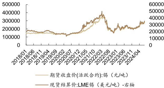
图 33：本周 SHFE 锡价下跌 0.6%,LME 锡价上涨 1.1%
