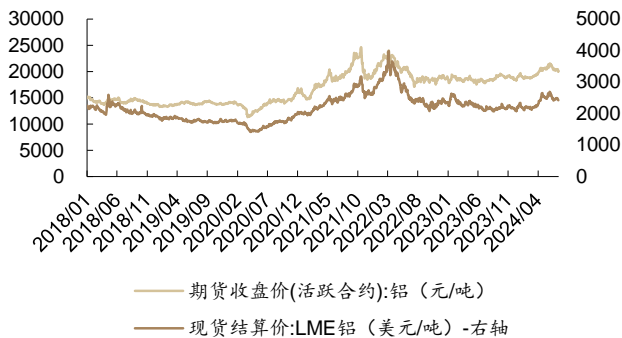
图 17: 本周 SHFE 铝价下跌 1.4%,LME 铝价下跌 2.9%
