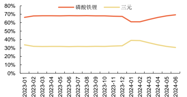
图10：磷酸铁锂和三元动力电池累计装车比例
