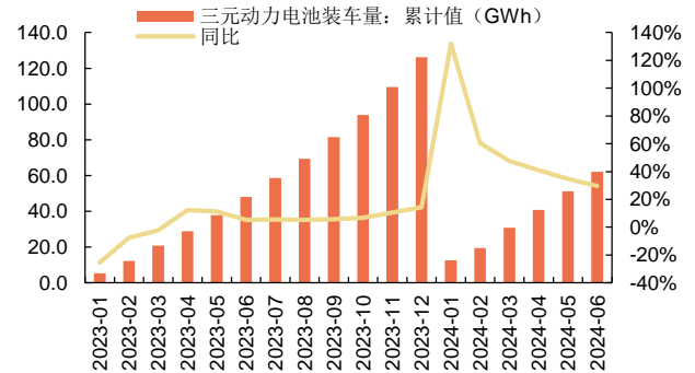
图8：三元动力电池装车量累计值及同比增速
