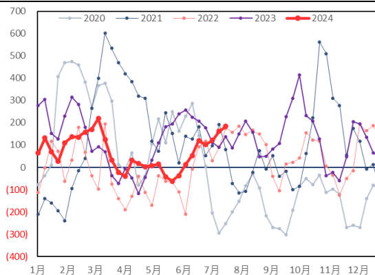
图 63: FDY 单吨净利润 (元/吨)
