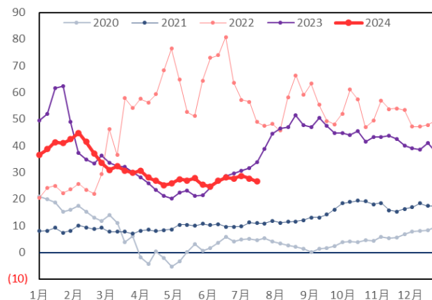
图 26: 原油、欧洲航煤价差 (美元/桶, 美元/桶)
