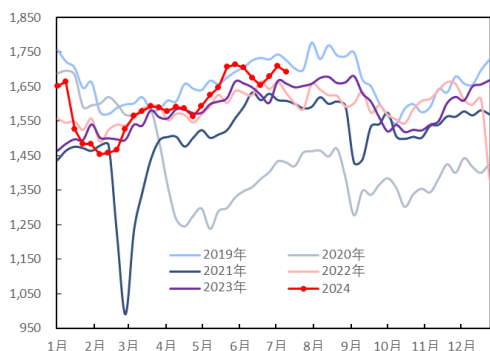
图 30: 美国炼厂原油加工量 (万桶/天)
