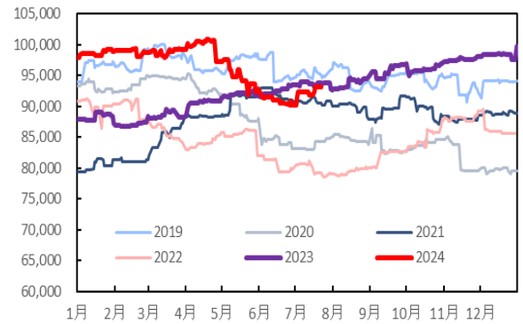
图 13：350 英尺+自升式钻井平台平均日费（美元/天）
