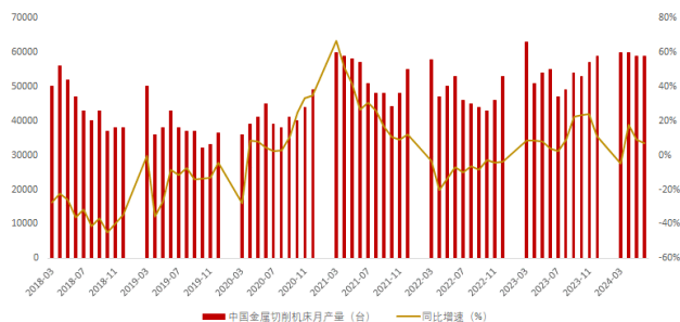
图 30：中国金属切削机床月产量及增速（台，%）
