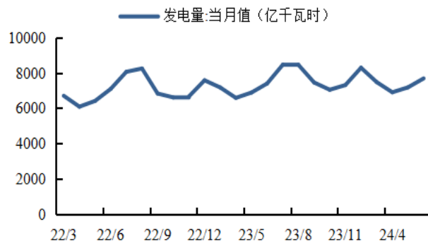
图16：6月发电 7685.20 亿千瓦时，环比上涨 7.06%
