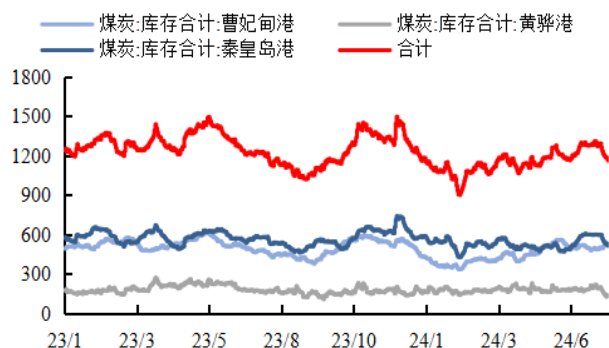
图11：7月三港合计煤炭库存量月环比下跌8.07%（万吨）
