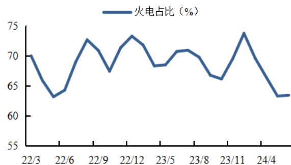
图18：6月火电占发电的比重达 63.37%，同比下降
