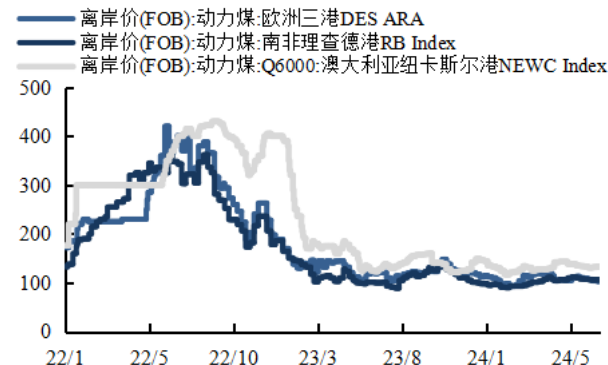
图4：7 月国际动力煤离岸价情况（美元/吨）
