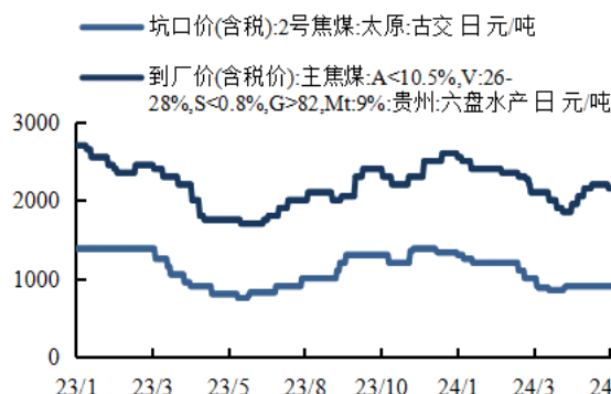
图22：7月太原和贵州炼焦煤价格
