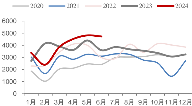
图表 62: 锡矿砂及精矿月度产量 (吨)
