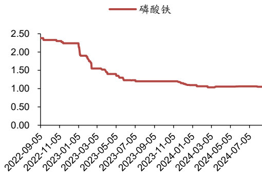
图 26: 磷酸铁价格走势 (万元/吨)
