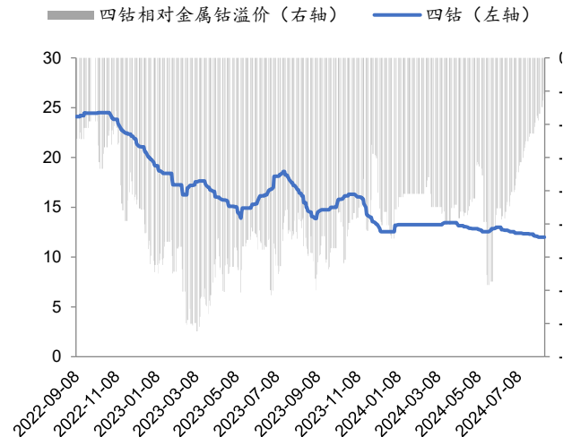
图 13: 四氧化三钴价格走势 (万元/吨)
