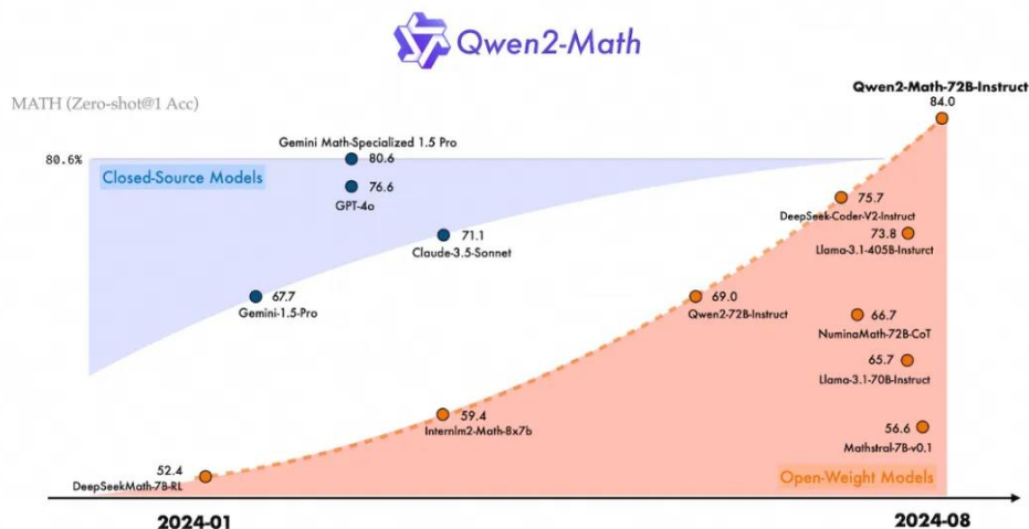
图 2：MATH 基准测评中，Qwen2-Math-72B-Instruct 取得 84% 准确率
