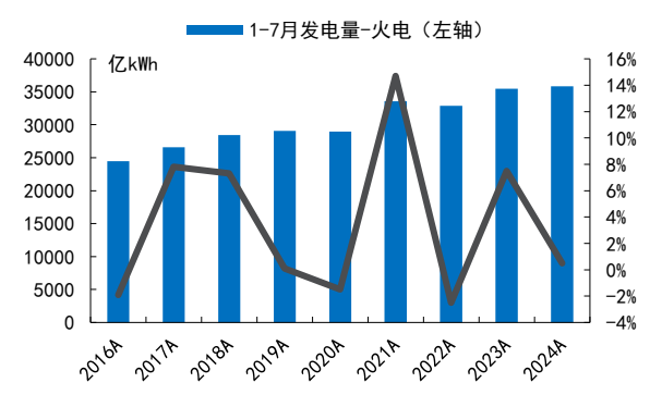
图表8: 24M1-7全国火电发电量同比增长0.5%
