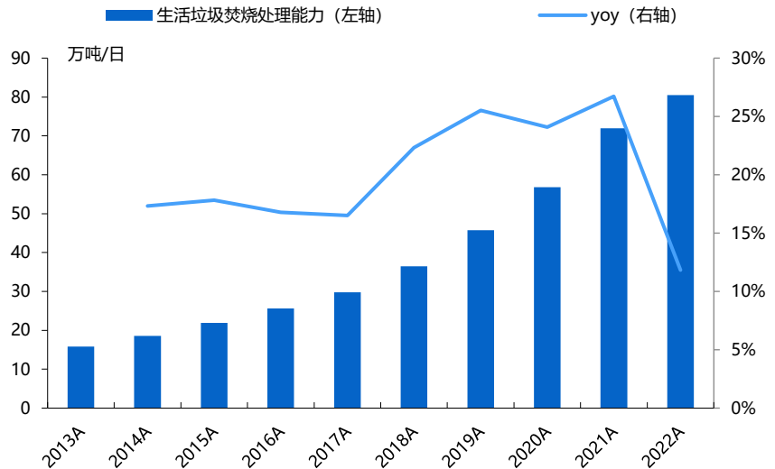
图表16: 2013-2022年，我国生活垃圾焚烧处理能力
