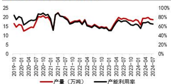
图：涤纶工业丝产量及产能利用率
