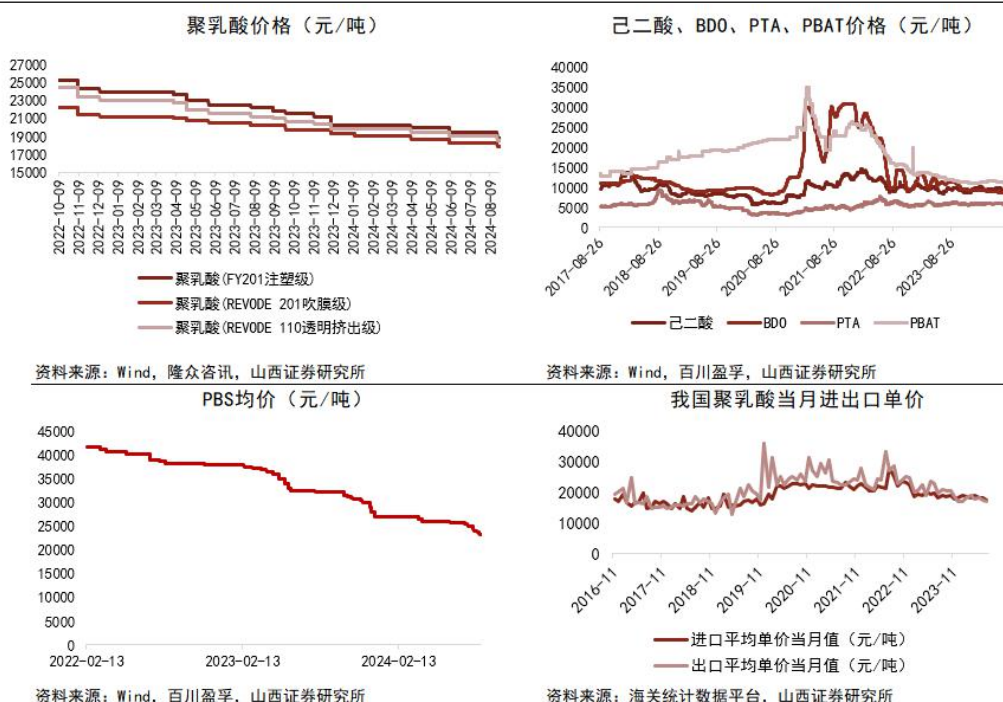
图 8：可降解塑料产业链价格情况
