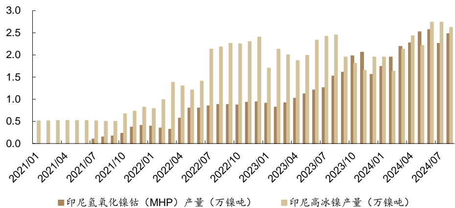
图 53: 2024 年 8 月, 印尼氢氧化镍钴 (MHP) 产量 2.48 万镍吨, 印尼高冰镍产量 2.62 万镍吨
