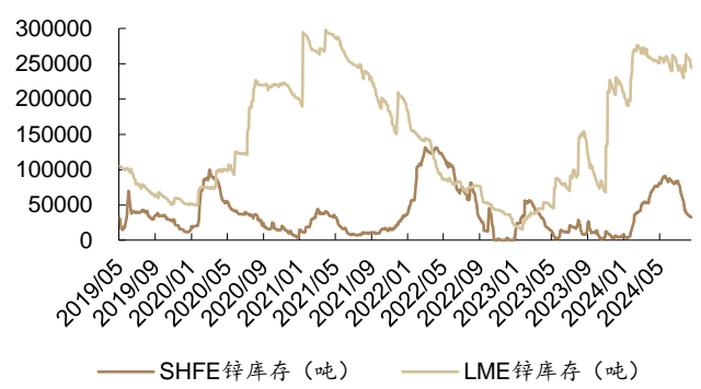
图 29: 本周 SHFE 锌库存减少 5.4%,LME 锌库存减少 4.4%
