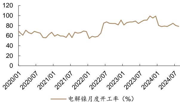
图 39: 2024 年 7 月, 电解镍月度开工率 80.03%
