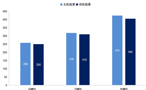
图12: 有无轮毂罩的燃油消耗
