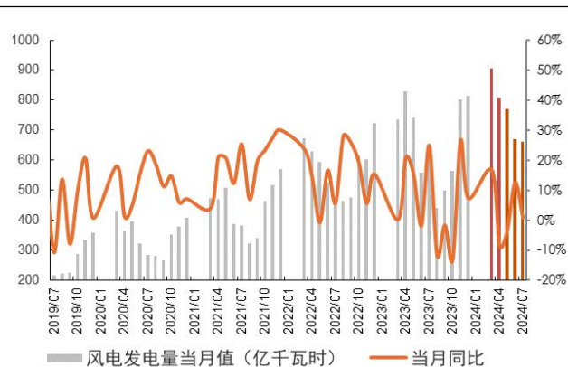
图 19：7 月风电发电量及增速
