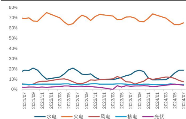
图 12：1-7 月分类型发电量占比
