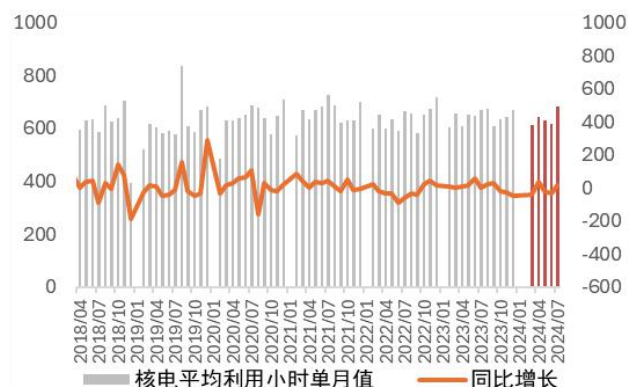
图 33：核电设备当月平均利用小时及同比
