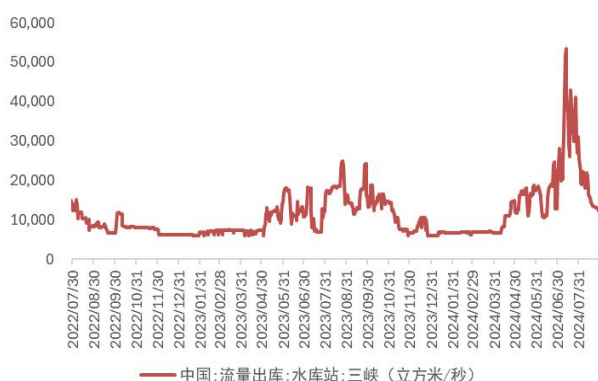
图45：三峡出库流量日行情（立方米/秒）
