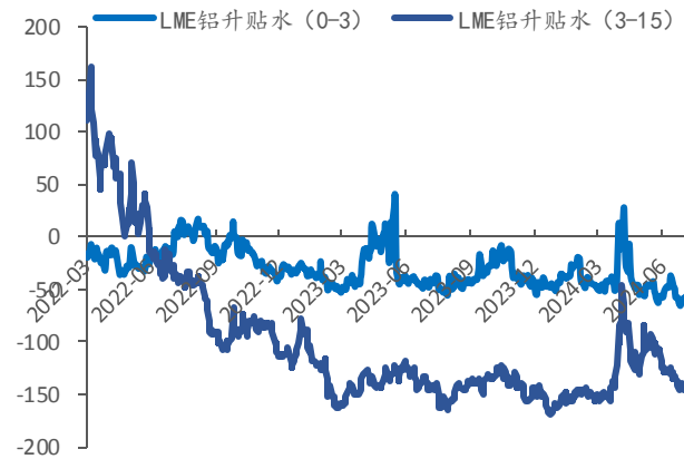
图表17: 铝期限结构 (美元/吨)
