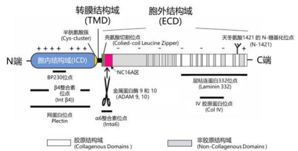
图7：XVII 型胶原蛋白上有多个非 G-X-Y 结构区
