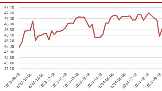
图 23：焦炭样本钢厂日均产量（万吨）
