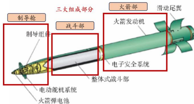
图表3: 远程火箭弹示意图
